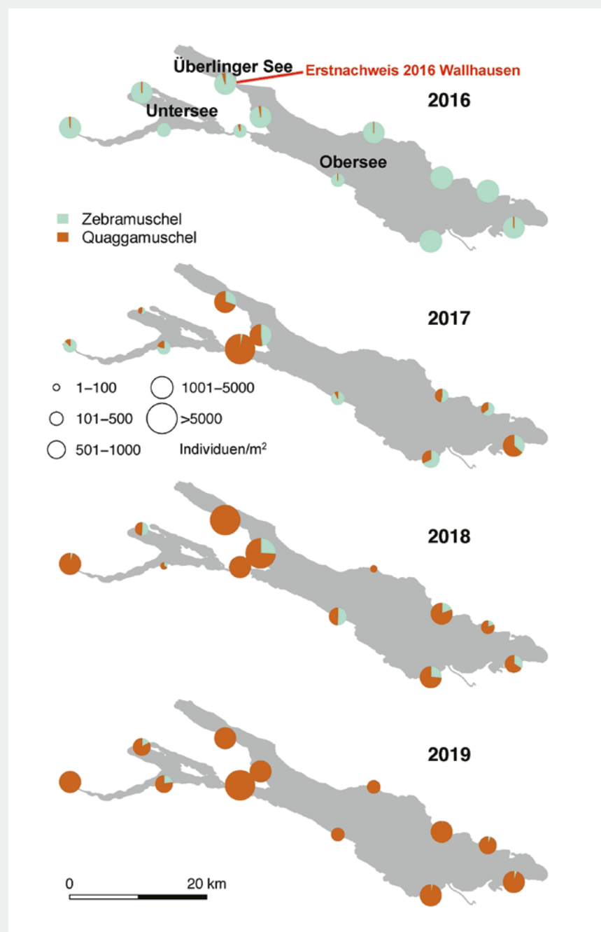
Fig. 2 Quantitative Schätzungen der relativen Häufigkeit von Quagga- (braun) und Zebamuschnen (grün) im Bodensee. Die Grösse der Tortendiagramme gibt die Anzahl der Muscheln an, die pro Quadratmeter an jeder Probenahmestelle gefunden wurden (aus: [4]).
